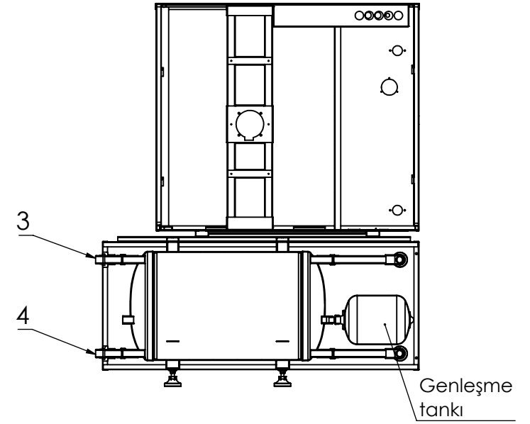
Ön görünüm
